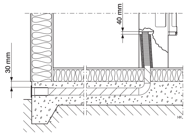
Durch Boden und Bodenplatte
