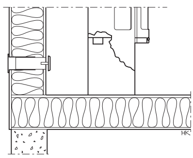
Indirekt durch die Außenwand
