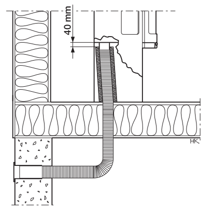
Durch Boden und Streifenfundament
